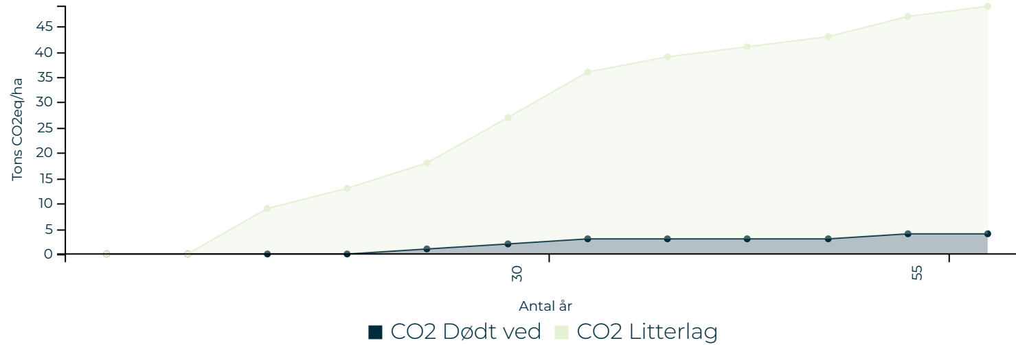
Figur 5: Estimeret udvikling af CO 2 i dødt ved og litterlag baseret på data fra Danmarks Skovstatistik.
